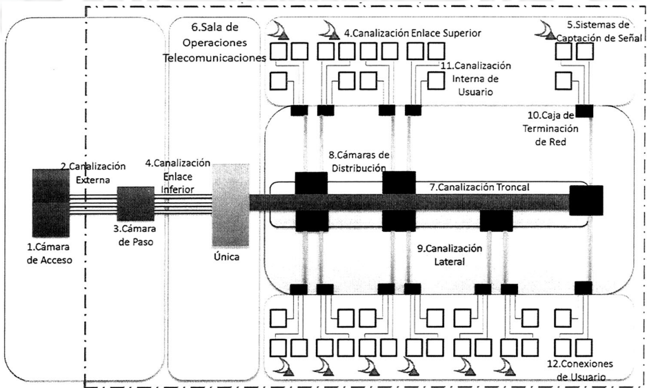
Red Interna de Telecomunicaciones (RIT) en Proyectos en Extensión (condominio y loteo)
